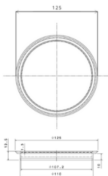
Couvercle (poids : 25g)
