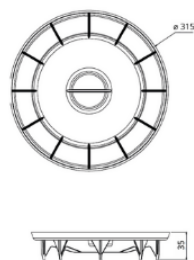
Couvercle (poids : 350g)
