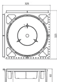
Base (poids : 300g)
