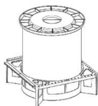
Ensemble (poids : 1100g) Réservation de Ø275mm après décoffrage. Pour passage de canalisation de Ø160, Ø200 ou Ø250 mm
